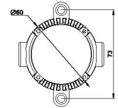
LPM-C2 单位/Unit : mm
